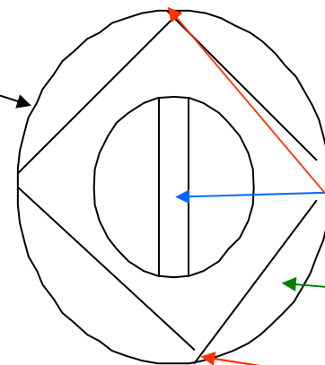
Vue du dessus de l'emboîtement d'un haut de bouteille carrée sur le corps d'une bouteille ronde
